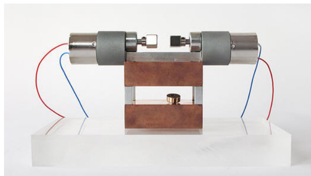
2 kubussen van het type W-12-N ( www.supermagnete.fr/dut/W-12-N )
