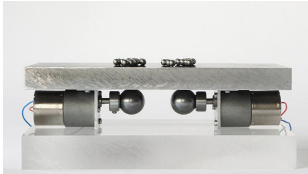
2 kogelmagneten van het type K-26-C ( www.supermagnete.fr/dut/K-26-C ) en 28 stalen kogels met een doorsnede van 3 mm
